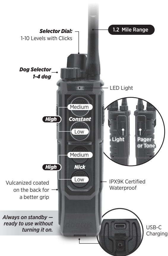
EDGE RT2 Transmitter
