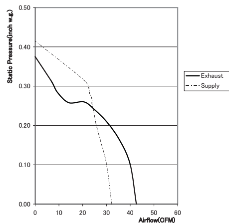
Fan Curve FV-04VE1
