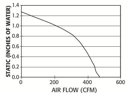
Fan Curve FV-40NLF1
