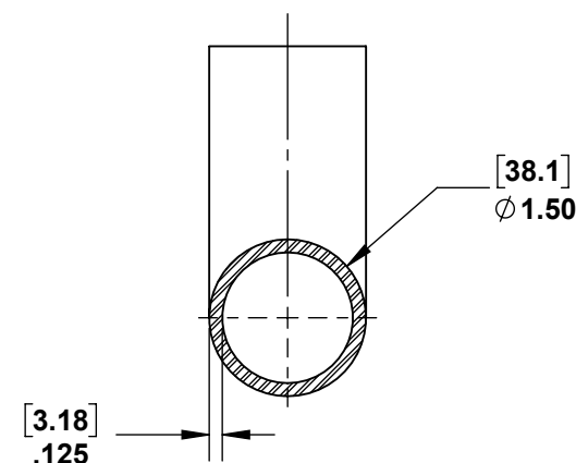
SECTION A-A SCALE 1 : 2
